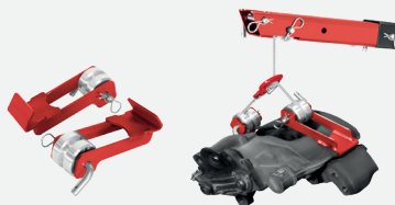
Zvedací hák pro brzdový třmen Max. 60 kg
